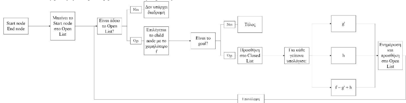
Σχήμα 23. Διάγραμμα ροής του AEA A*
